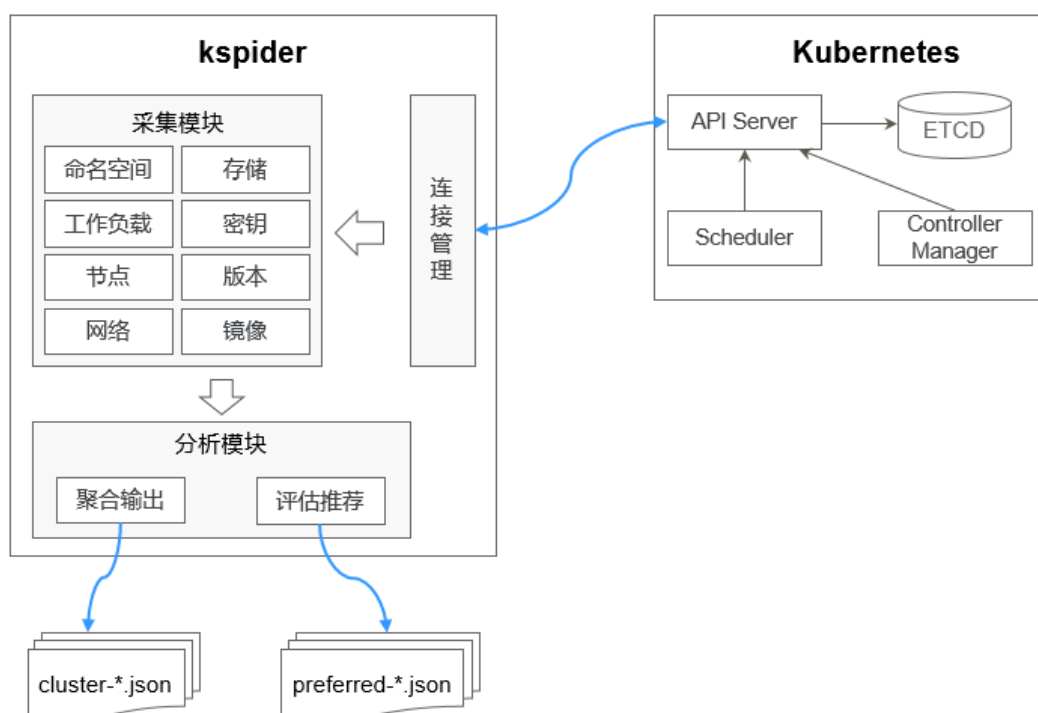
图 12-7 kspider 架构
