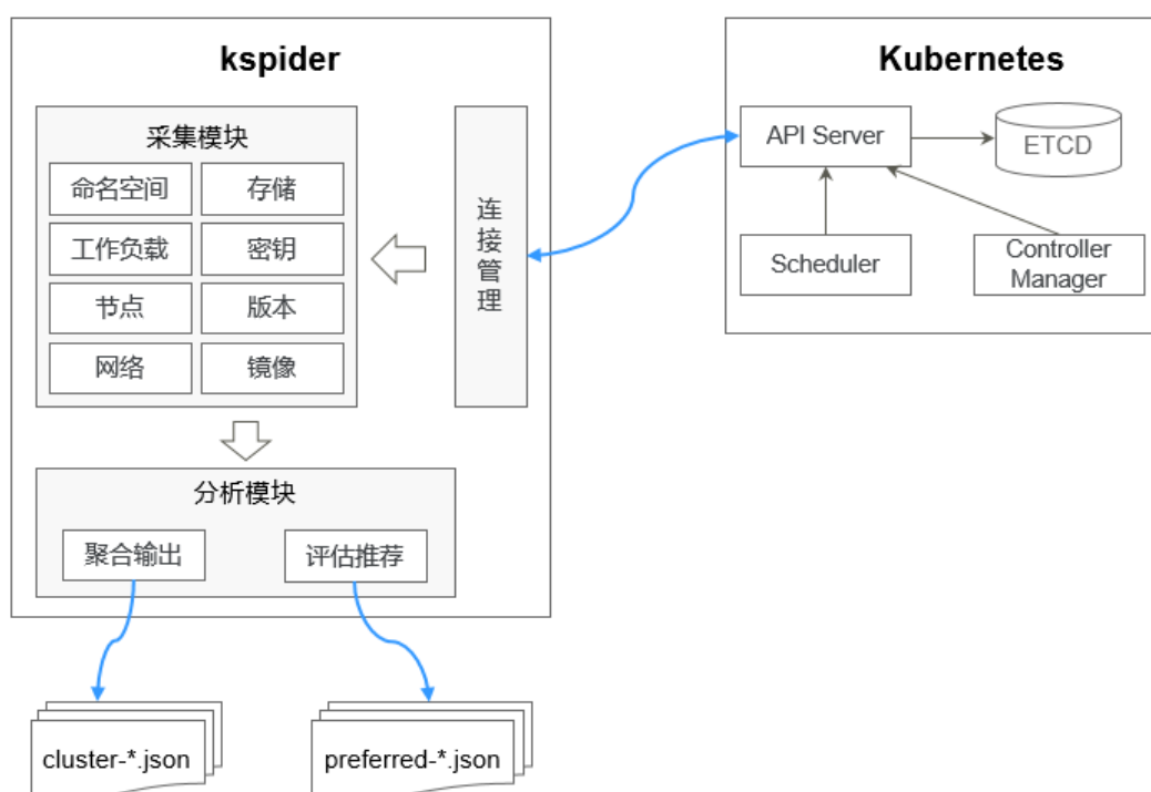
图 12-2 kspider 架构
