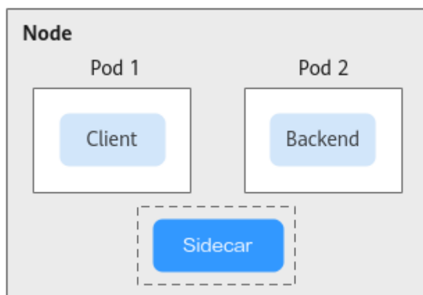
图 8-5 node-proxy
