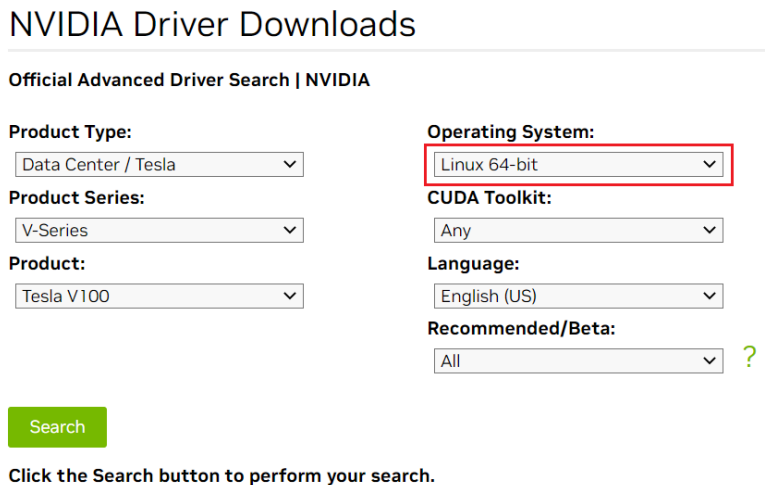
图 1-50 参数选择
