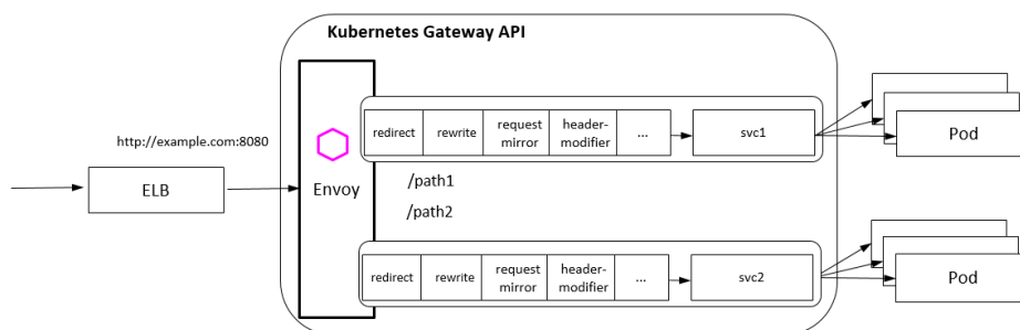
图 8-8 服务网关
