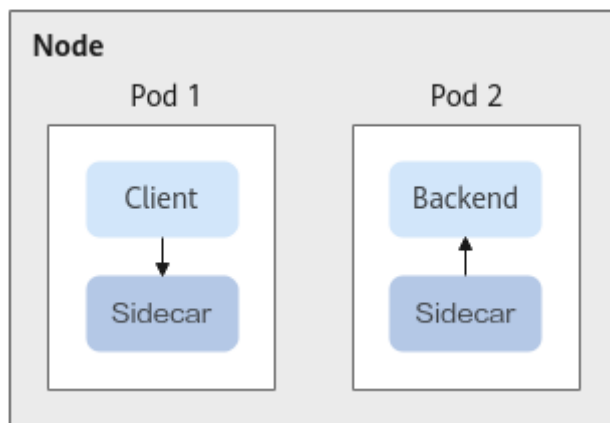
图 8-4 sidecar-proxy
