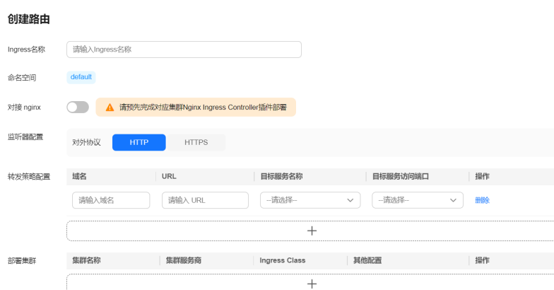
图 3-30 创建路由
