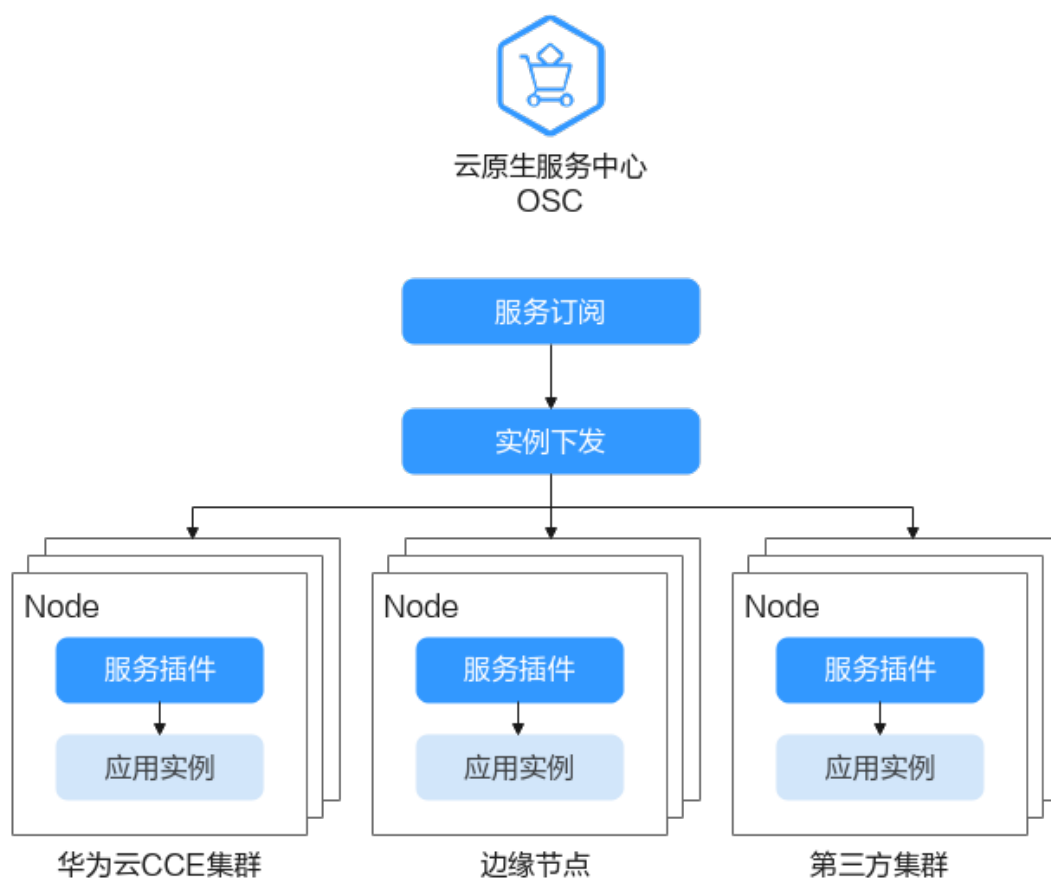
图 11-1 OSC 流程示意图
