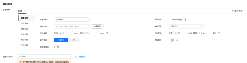
图 1-36 容器配置
