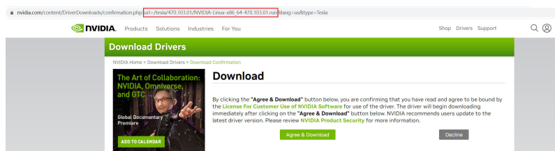
图 1-52 获取链接
