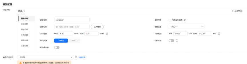
图 1-38 容器配置
